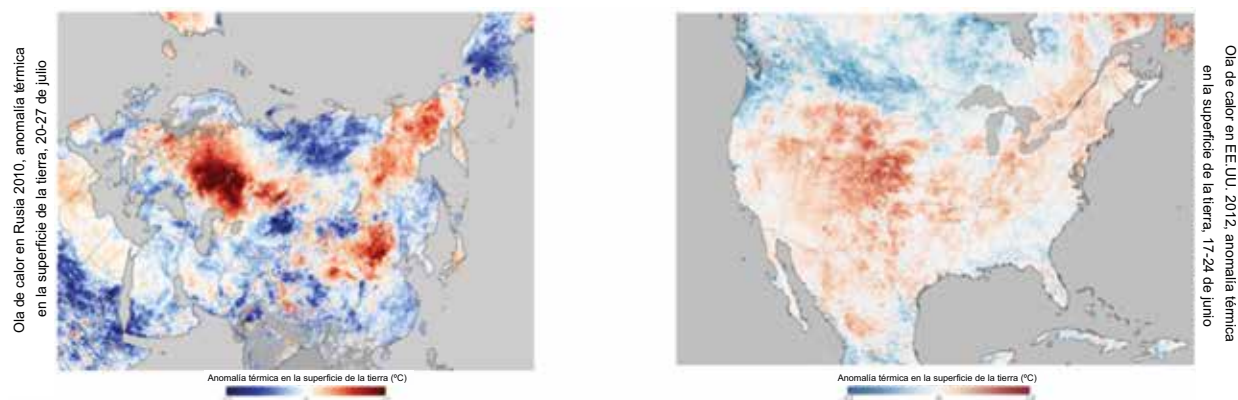
Figura 14: Oleadas de calor anormales en Rusia (2010) y Estados Unidos (2012), según medición satelital.
