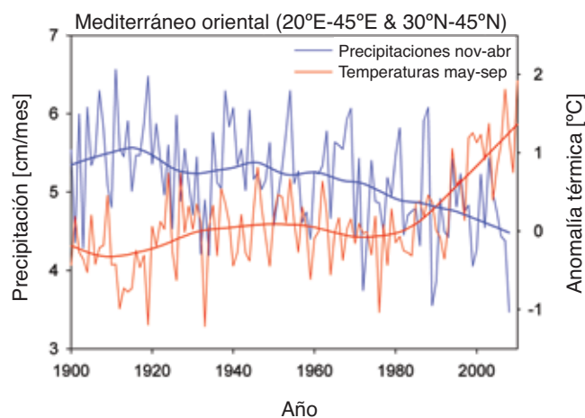
Figura 19: Precipitaciones invernales observadas (azul) que más contribuyen al presupuesto hídrico anual y temperaturas estivales (rojas) más importantes con respecto al secado por evaporación, con su tendencia a largo plazo para la región del Mediterráneo oriental.
