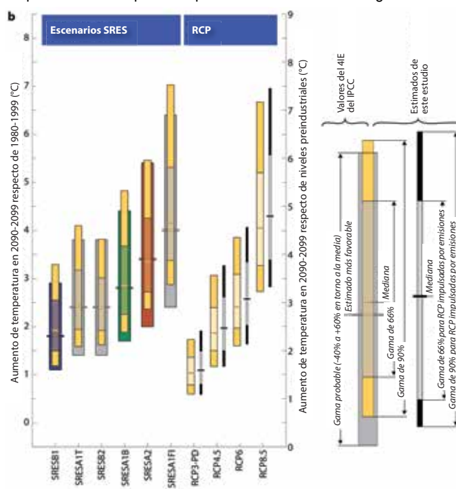
Figura 20: Estimados probabilísticos de la temperatura para escenarios de IPCC antiguos (SRES) y nuevos (RCP). Dependiendo de la trayectoria global de emisiones seguida, el umbral del aumento de temperatura de 4°C podría superarse antes de fines de siglo.
