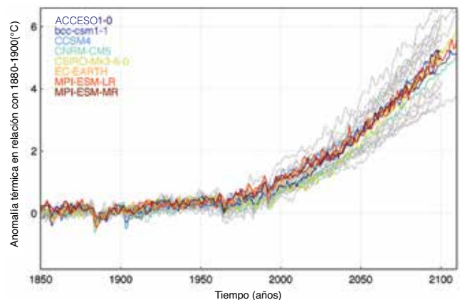
Figura 24: Simulación de anomalías térmicas históricas y promedios globales del siglo XXI en comparación con el período preindustrial (1880–1900) para 24 modelos CMIP5 sobre la base del escenario de la RCP8,5. Las curvas coloreadas (y etiquetadas) muestran aquellas simulaciones que alcanzan un calentamiento promedio mundial de 4°C a 5°C en 2080-2100 por sobre la era preindustrial, las que se utilizan para realizar análisis adicionales.
