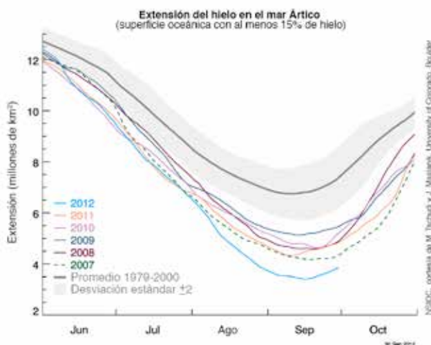
Figura 13: Panel izquierdo: Extensión del hielo en el mar Ártico entre 2007–2012; el promedio entre 1979–2000 está en gris oscuro; el sombreado en gris claro representa dos desviaciones estándar. Panel derecho: Variaciones plurianuales en el hielo desde 1983 hasta 2012.
