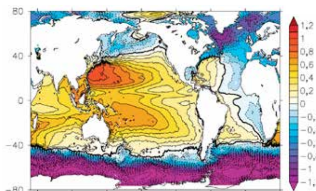
Figura 30: Topografía dinámica del nivel del mar actual. Esta figura muestra las desviaciones del nivel del mar de la geoide (es decir, la superficie oceánica determinada por el campo gravitacional, si los océanos estuvieran en reposo). El nivel del mar que está por sobre el promedio se muestra en naranja/rojo, mientras que si está bajo el promedio, en azul/violeta. Las líneas del contorno indican intervalos de 10 centímetros. Esta “topografía dinámica” refleja el equilibrio entre la pendiente de la superficie y los sistemas de corrientes oceánicas. Un aspecto digno de mencionar es el nivel del mar bajo el promedio a lo largo de la costa nororiental de Estados Unidos asociada a la corriente del Golfo. Se proyecta que el cambio climático provocará una desaceleración de la corriente del Golfo durante el siglo XXI y el correspondiente aplanamiento de la superficie del océano. A su vez, este efecto por sí solo llevaría al alza del nivel del mar en esa zona. Sin embargo, es importante destacar que no existe un vínculo sistemático entre la topografía dinámica actual (mostrada en esta figura) y el incremento en el nivel del mar a futuro en virtud del cambio climático.
