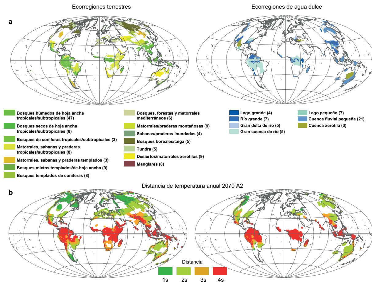
Figura 36: Distribución de la temperatura mensual proyectada para 2070 (calentamiento de 2,9°C) en los componentes terrestres y de agua dulce de Global 200 de WWF. (A) Distribución de 132 ecosistemas terrestres y 53 de agua dulce, agrupados por biomas. (B) Distancia promedio (medida en número de desviaciones estándar de la media) de las temperaturas mensuales del siglo XXI desde aquella del período de base (1961–1990).
