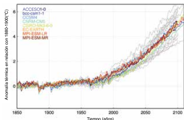
Figura A2.1: Anormalidades simuladas de la temperatura media global histórica y del siglo XXI, en comparación con el período preindustrial (1880–1900), para 24 modelos CMIP5 basados en el escenario RCP8,5. Las curvas coloreadas (y rotuladas) muestran que dichas simulaciones alcanzan un calentamiento medio global de 4°C–5°C por sobre los niveles preindustriales en 2080–2100, las que se utilizan para análisis adicionales.
