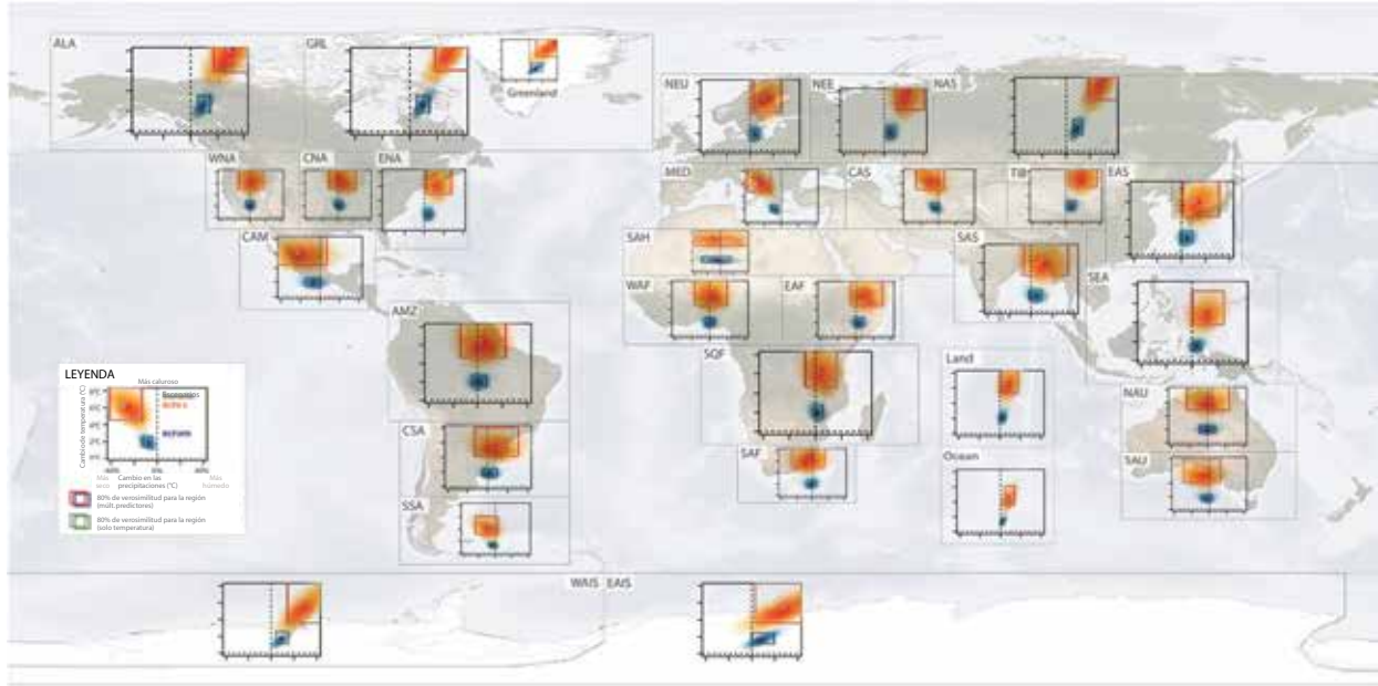
Figura 23: Correlación entre calentamiento regional y cambios en el régimen de precipitaciones en la forma de distribuciones conjuntas de las temperaturas medias regionales y cambios en las precipitaciones en 2100, para los escenarios RCP3-PD (azul) y RCP8,5 (naranja). Este último es superior al calentamiento global de 4°C en 2100. La distribución muestra la incertidumbre en la relación entre calentamiento y precipitación para 20 de los MCGAO utilizados en el 4IE del IPCC y considera los efectos significativos de los aerosoles en los patrones regionales. Los rectángulos indican el 80% interior de las distribuciones marginales y el etiquetado de los ejes es idéntico en todos los subpaneles y en la leyenda. Las definiciones de las regiones se basan en Giorgi y Bi (2005) y se utilizan frecuentemente para describir cambios climáticos a gran escala en zonas terrestres. Aquí se encuentran modificados por los indicados para los mantos de hielo de la Antártica occidental y oriental, separados por la Cordillera Transantártica.
