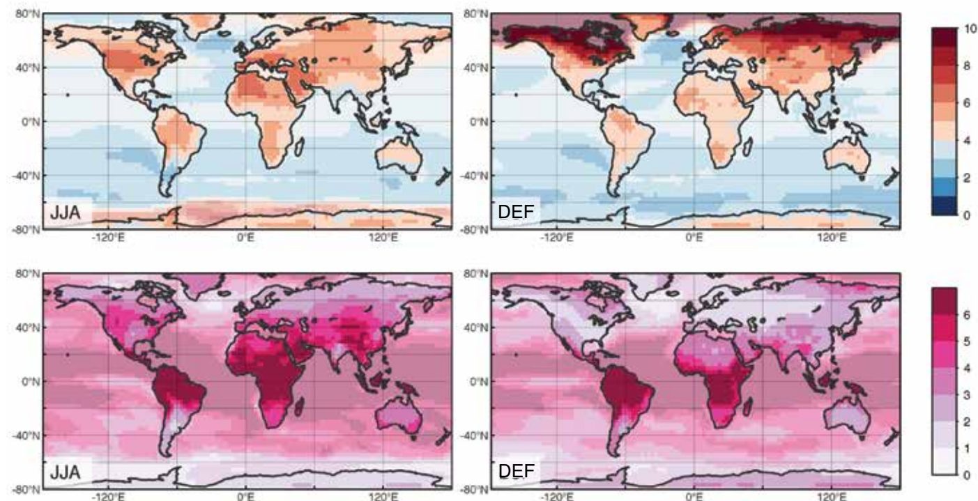
Figura 33: Media de múltiples modelos del calentamiento mensual durante el siglo XXI (2080–2100 con respecto al presente) para los meses de junio a agosto (izquierda) y diciembre a febrero (derecha) en unidades de grados Celsius (arriba) y desviación estándar de la temperatura local (abajo). La intensidad de la escala de color se atenuó sobre el océano para que se distinga mejor.
