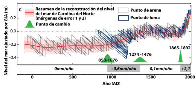
Figura 8: Registro del nivel del mar en Carolina del Norte reconstruido durante los últimos 2.000 años. El período posterior a fines del siglo XIX muestra claramente el aumento del nivel de los océanos inducido por el hombre.
