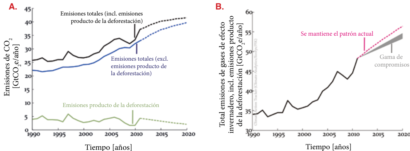
Figura 2: Emisiones globales de CO 2 (a) y totales de gases de efecto invernadero (b), tanto históricas (líneas continuas) como proyectadas (líneas quebradas). Fuente de datos de CO 2 : línea base PRIMAP4BIS a ; y fuente de datos sobre gases de efecto invernadero: Climate Action Tracker b . Las trayectorias globales incluyen emisiones del transporte internacional. El rango de las promesas en (b) proviene de las actuales mejores estimaciones de los compromisos establecidos por los países y van desde: ambición mínima, promesas incondicionales y reglas permisivas hasta ambición máxima, promesas condicionadas y reglas más estrictas.
