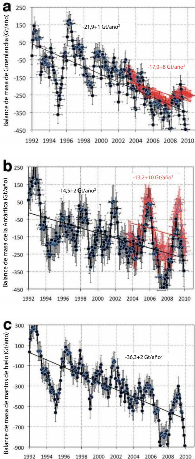
Figura 9: Balance total de masa de mantos de hielo, dM/dt , entre 1992 y 2010, para (a) Groenlandia, (b) Antártica y (c) suma de Groenlandia y Antártica, en Gt/año según el método de cálculo de masa (MBM) (círculo negro sólido) y la gravedad variable-en el tiempo GRACE (triángulo rojo sólido), con barras de error asociadas.
