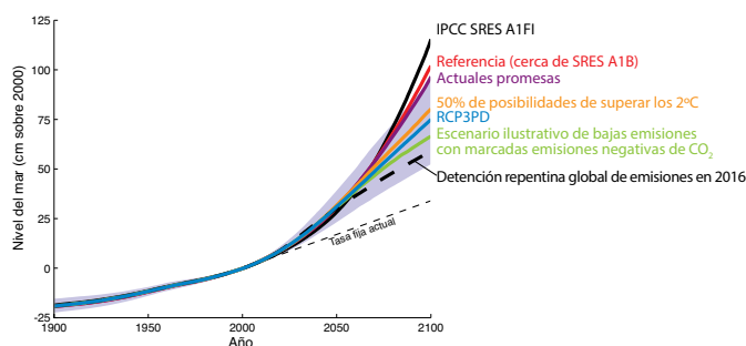
Figura 28: Tal como en la figura 22, pero para el aumento medio global del nivel del mar usando un método parcialmente empírico. La tasa actual indicativa/fija de 3,3 mm.año -1 es la tasa media satelital del período 1993–2007 (Cazenave y Llovel, 2010). Estimaciones medias a partir de proyecciones probabilísticas. Ver más detalles en Schaeffer et al. (2012) y en la leyenda de la Figura 22.
