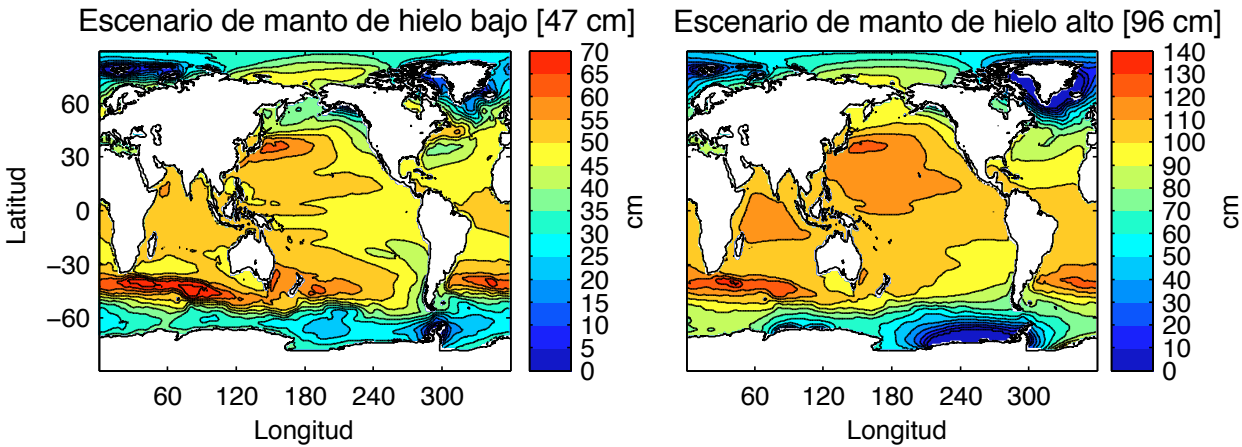
Figura A1.1: Proyección regional del nivel del mar para el escenario de aporte más bajo (izquierda) y más alto (derecha) del manto de hielo. Los números en paréntesis denotan el valor correspondiente de la media global del aumento en el nivel del mar, de 47 centímetros y 96 centímetros, respectivamente.
