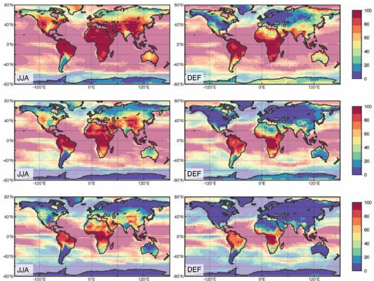
Figura 34: Media de múltiples modelos del porcentaje de meses durante 2080-2100 que serán más cálidos que 3-(arriba), 4 (al medio) y 5-sigma (abajo), en relación con la climatología actual, para los meses de junio a agosto (izquierda) y diciembre a febrero (derecha). La intensidad de la escala de color se atenuó sobre el océano para que se distinga mejor.
