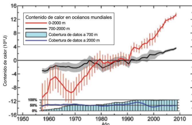
Figura 4: Aumento del contenido total de calor en el mar desde la superficie hasta los 2.000 metros, sobre la base de análisis en curso durante cinco años. El período de referencia es 1955-2006. La línea negra muestra el contenido creciente de calor a cierta profundidad (700 a 2.000 metros) e ilustra una tendencia considerable y en alza, mientras que la mayor parte del calor se queda en los primeros 700 metros del océano. Las barras verticales y la zona sombreada representan una desviación estándar de \pm 2 respecto de la estimación de cinco años para las respectivas profundidades.
