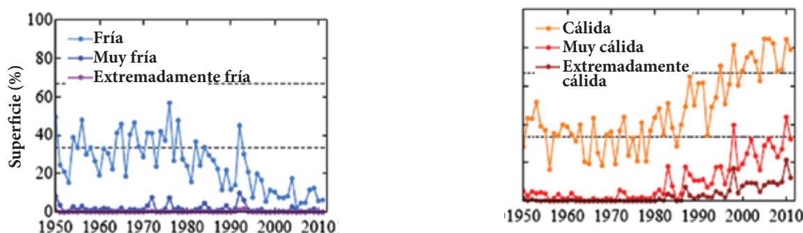
Figura 18: Superficie de tierra del hemisferio norte afectada por temperaturas estivales (panel izquierdo) frías ( < -0,43\sigma ), muy frías ( < -2\sigma ), extremadamente frías ( < -3\sigma ) y (panel derecho) calurosas ( > 0,43\sigma ), muy calurosas ( > 2\sigma ) y extremadamente calurosas ( > 3\sigma ).
