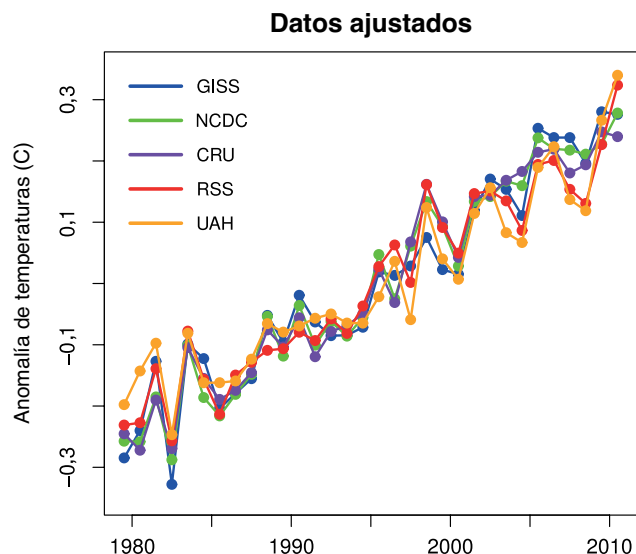
Figura 3: Datos sobre temperatura de diferentes fuentes (GISS: Goddard Institute for Space Studies GISS de la NASA; NCDC: NOAA National Climate Data Center; CRU: Hadley Center/Climate Research Unit, RU; RSS: datos de sistemas de detección remota; UAH: Universidad de Alabama en Huntsville) corregidos según la variabilidad de la temperatura a corto plazo. Cuando los datos se ajustan para eliminar el impacto estimado de factores conocidos en las variaciones de temperatura a corto plazo (corriente de El Niño, aerosoles volcánicos y variabilidad solar), la señal de calentamiento global es evidente.
