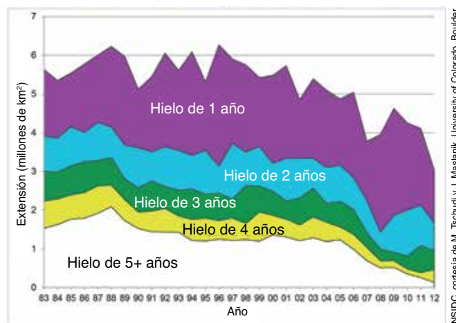
Figura 13: Panel izquierdo: Extensión del hielo en el mar Ártico entre 2007–2012; el promedio entre 1979–2000 está en gris oscuro; el sombreado en gris claro representa dos desviaciones estándar. Panel derecho: Variaciones plurianuales en el hielo desde 1983 hasta 2012.
