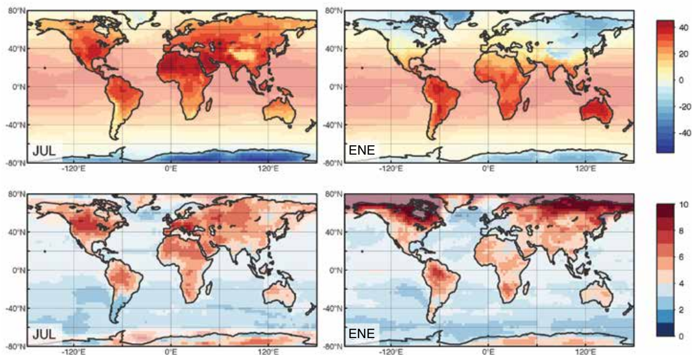
Figura 35: Compilación de las medias (de múltiples modelos) de la temperatura mensual extrema más cálida en cada ubicación durante 2080–2100 entre los meses de julio (izquierda) y enero (derecha) en temperaturas absolutas (arriba) y anomalías comparadas con la temperatura mensual más extrema simulada para la actualidad (abajo). La intensidad de la escala de color se atenuó sobre el océano para que se distinga mejor.
