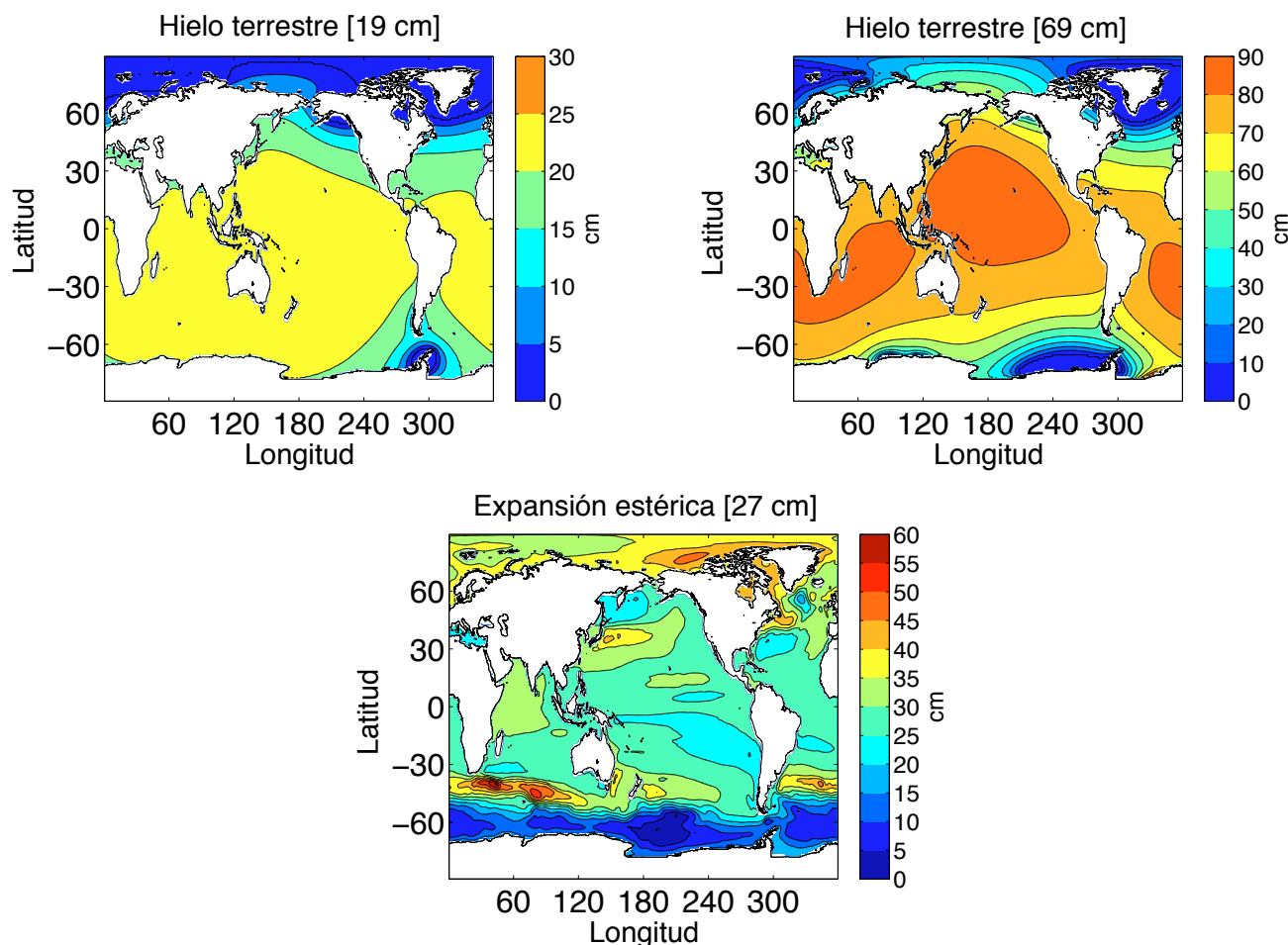
Figura A1.3: Aportes individuales al aumento del nivel del mar en 2100 en un mundo con 4°C más: contribución del hielo de la tierra (glaciares de montaña y casquetes de hielo + mantos de hielo) en el escenario de aporte más bajo (arriba-izquierda) y más alto (arriba-derecha) del manto de hielo; expansión térmica media global más la dinámica de los cambios en el nivel del mar (denominados en conjunto “expansión estérica”) (abajo izquierda). Los promedios mundiales se indican en paréntesis. El sombreado gris indica bajas en el nivel del mar (valores negativos). Vale la pena observar que los autores no excluyen los beneficios más altos de la mitigación, en particular, el posible (pero incierto) quiebre de los puntos de inflexión respecto del colapso de los mantos de hielo que podrían profundizar los efectos de un mundo con 4°C más en comparación con uno con 2°C más.
