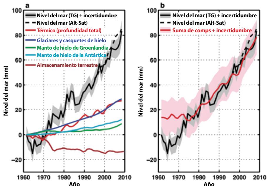
Figura 6: Panel izquierdo (a): aportes del hielo de la tierra (glaciares de montaña y casquetes de hielo y los mantos de hielo de Groenlandia y la Antártica), aumento termostérico del nivel del mar y almacenamiento en la tierra (efectos netos de extracción de aguas subterráneas y construcción de represas), así como observaciones de mareógrafos (desde 1961) y observaciones satelitales (desde 1993). Panel derecho (b): la suma de los aportes individuales se aproxima al alza observado en el nivel del mar desde los años setenta. Los vacíos en el período anterior podrían ser el resultado de errores en las observaciones.
