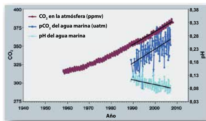
Figura 11: Cambios observados en la acidez del océano (pH) comparados con la concentración de dióxido de carbono disuelto en el agua marina ( \text{pCO}_2 ), junto con el registro de \text{CO}_2 en la atmósfera desde 1956. Una disminución en el pH indica un aumento en la acidez.
