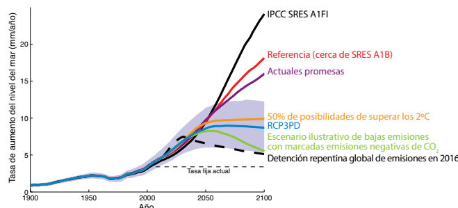
Figura 29: Tal como en la figura 22, pero para la tasa anual de aumento del nivel de mar medio global. La tasa actual indicativa/fija de 3,3 mm.año -1 es la tasa media satelital 1993–2007 (Cazenave y Llovel, 2010). Estimaciones medias a partir de proyecciones probabilísticas (ver más detalles en Schaeffer et al., 2012, y en la leyenda de la figura 22).
